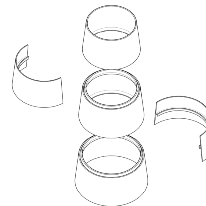
Esplosione elemento nelle sue 5 parti, vista e forma concettuale e relativo ingombro nello spazio. Corpo e pannelli in ceramica; possibile opzione riguarda l'uso di altri materiali per i pannelli rotanti esterni, con leghe di alluminio o plastiche
